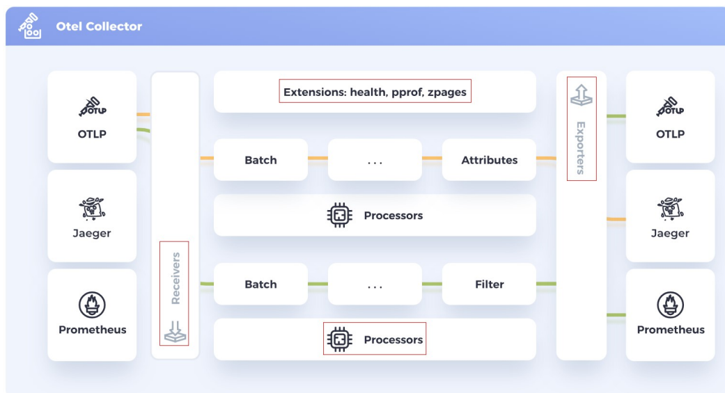
图 1-1 otel-collector 架构图
